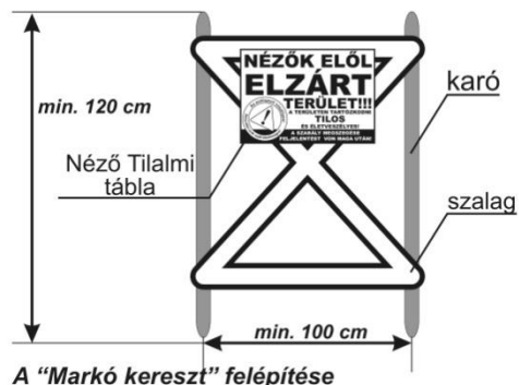
A "Markó kereszt" felépítése
